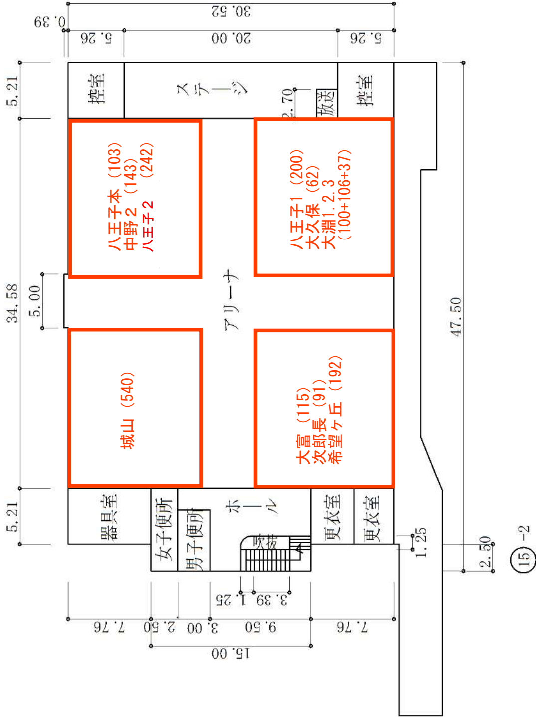
2階平面図
