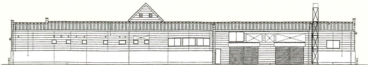
西側立面図
