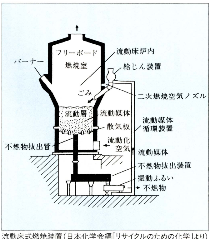
流動床式燃焼装置(日本化学会編「リサイクルのための化学」より)
