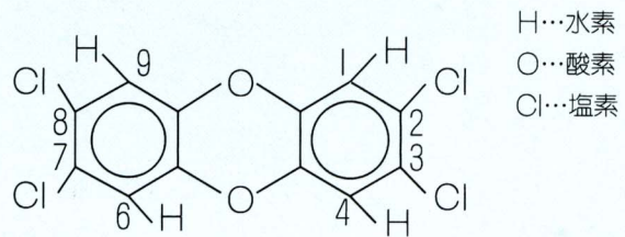
2,3,7,8-四塩化ダイオキシンの化学構造式
