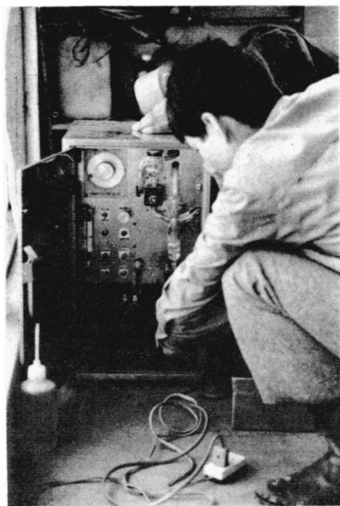
硫化水素ガス測定状況
