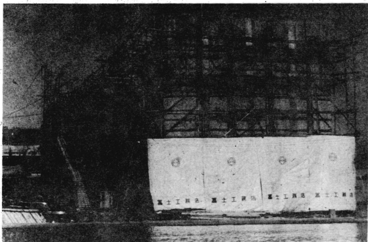
写真 第二小学校鉄筋コンクリート三階建5月31日完成予定
